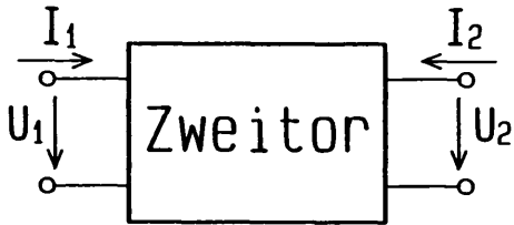
Abb.1 Vorzeichenkonvention für die elektrischen Klemmengrößen
